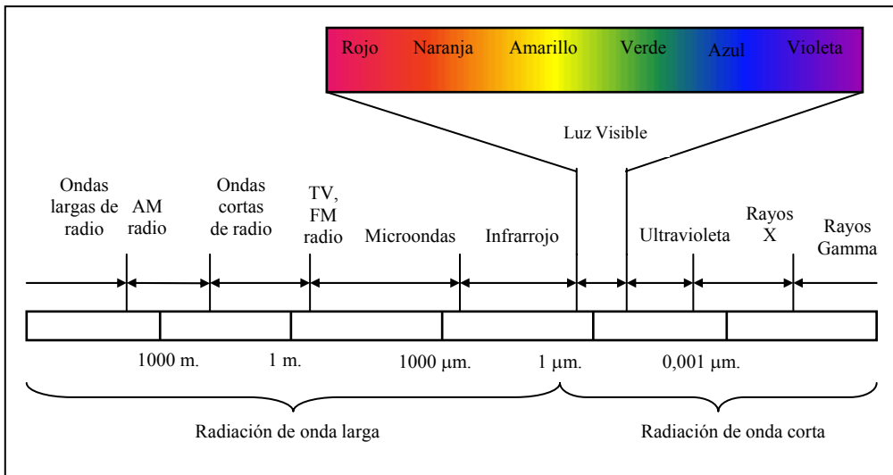
Figura 1. Espectro electromagnético .
